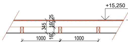
ŘEZ PODÉLNÝ
