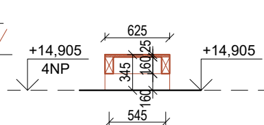
ŘEZ PŘÍČNÝ
